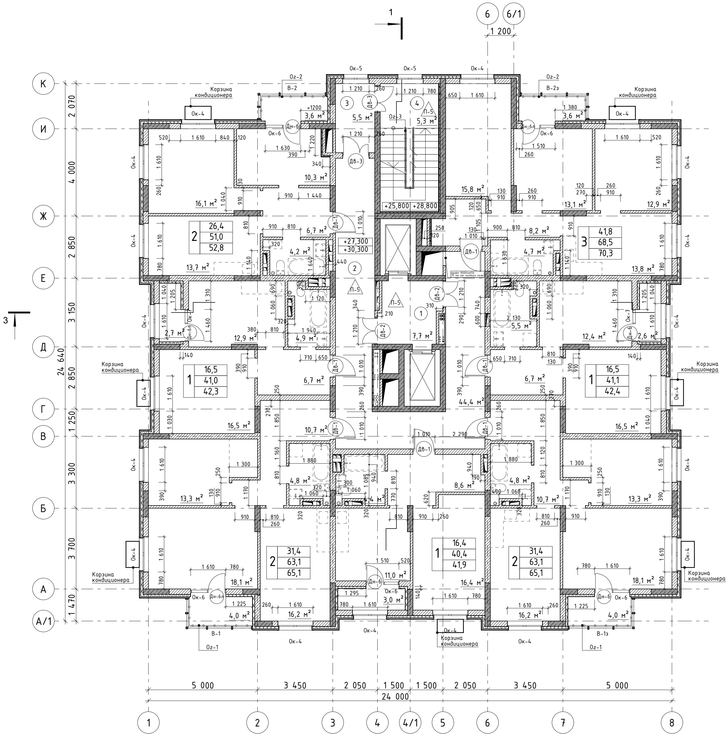
План на отм.+27,300;+30,300 М1:100
