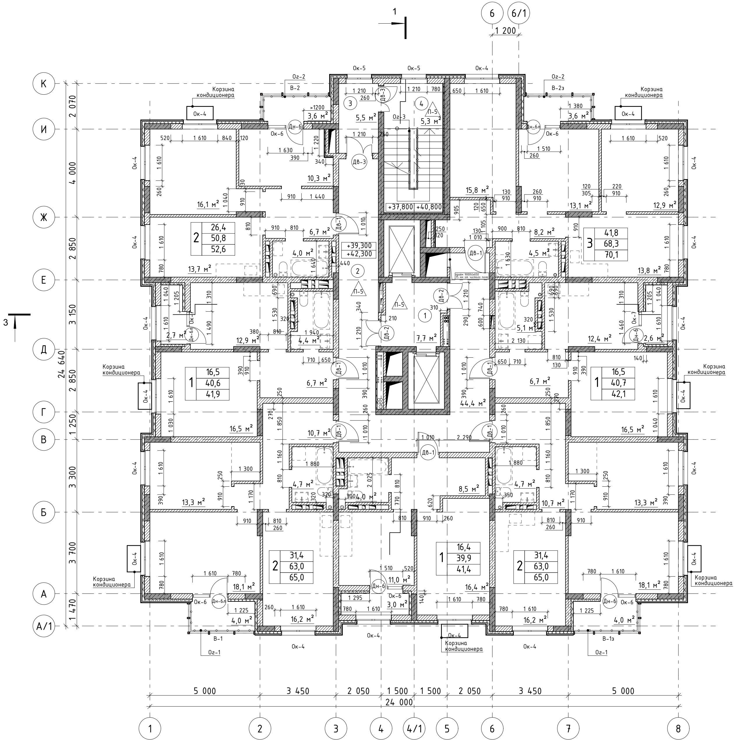
План на отм.+39,300;+42,300 М1:100
