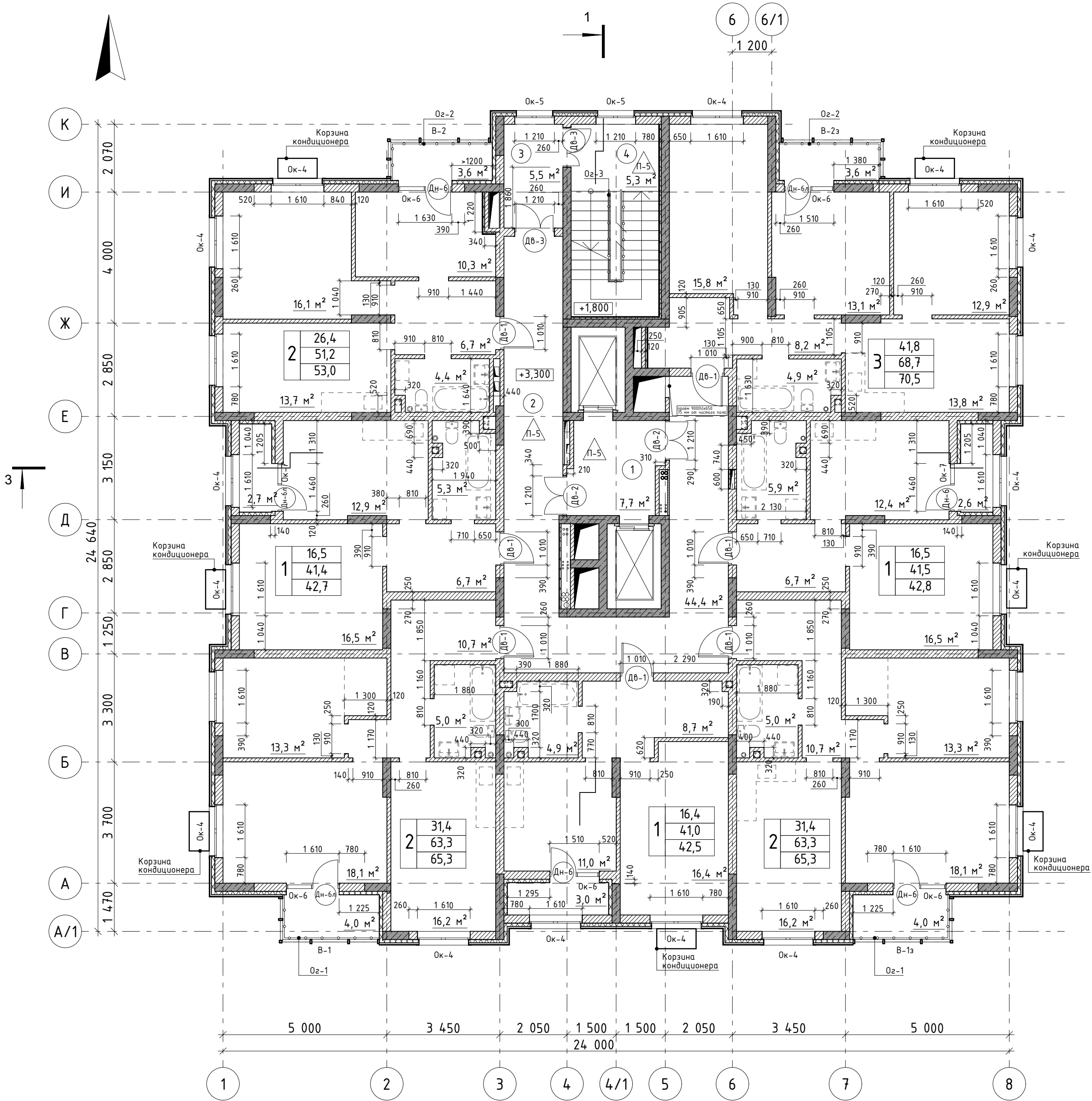
План на отм.+3,300 М1:100
